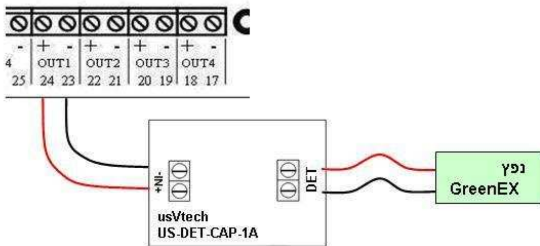
סכמת חיבורים כרטיס מתאם כיבוי
