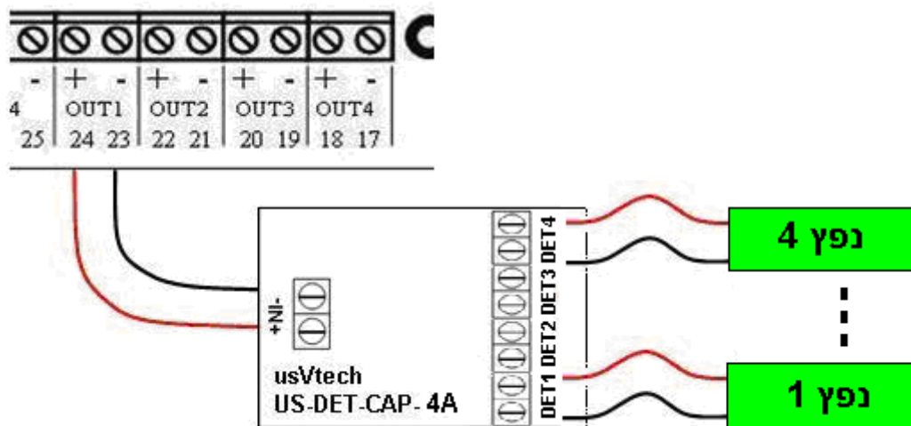
סכמת חיבורים כרטיס מתאם כיבוי
