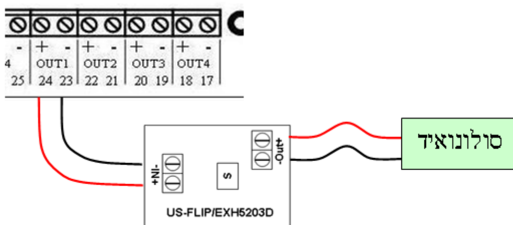
סכמת חיבורים כרטיס מתאם עבור כיבוי באמצעות סולנואיד
