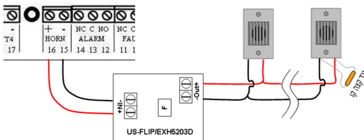
סכמת חיבורים כרטיס מהפך
